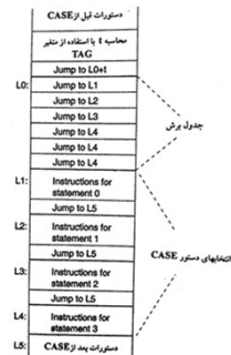
شکل ۷-۱ پیاده سازی جدول پرش دستور case
