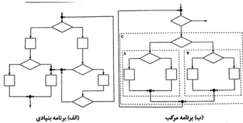
شکل ۸-۸ فلوچارتها
